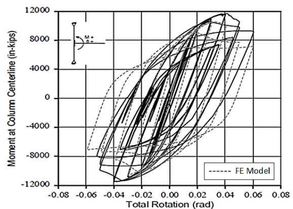
شکل (۵): مقایسه منحنی ممان-چرخش مدل اتصال با نتیجه آزمایشگاهی
