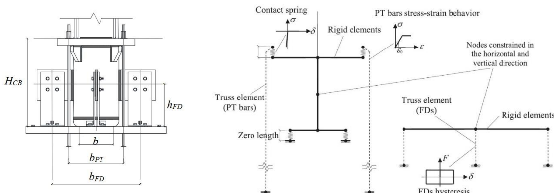
شکل ۶- مدل پای ستون گهواره‌ای در نرم‌افزار Opensees [۱۰]
