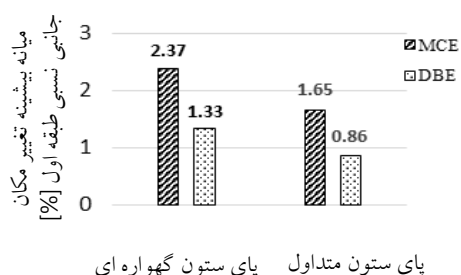
شکل ۱۴- مقادیر میانه بیشینه تغییر مکان جانبی نسبی طبقه اول
