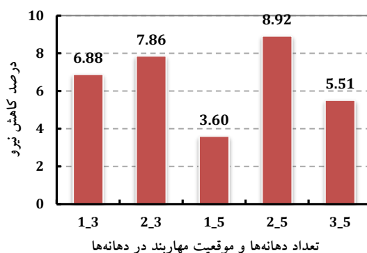
شکل ۷- درصد کاهش برش پایه در قاب‌های سه طبقه با سه و پنج دهانه با مهاربند قطری با مقطع کاهش یافته به نسبت قاب با مهاربند قطری معمولی در دهانه‌های مختلف
