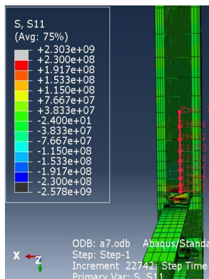
شکل ۲۶- تنش‌های پسماند در راستای محور x ها برای اتصال ورق روسری به ستون
