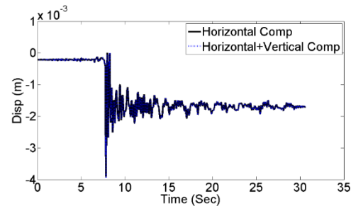
شکل ۲۵- تاریخچه جابجایی گره مبناي قاب ۴ طبقه تحت شتاب نگاشت Taiwan Smart 1 در سناریوی S1
