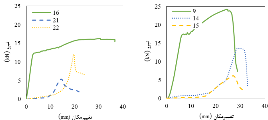
شکل ۱۷- بررسی میزان پوشش‌های متفاوت در نتایج نمونه‌ها
