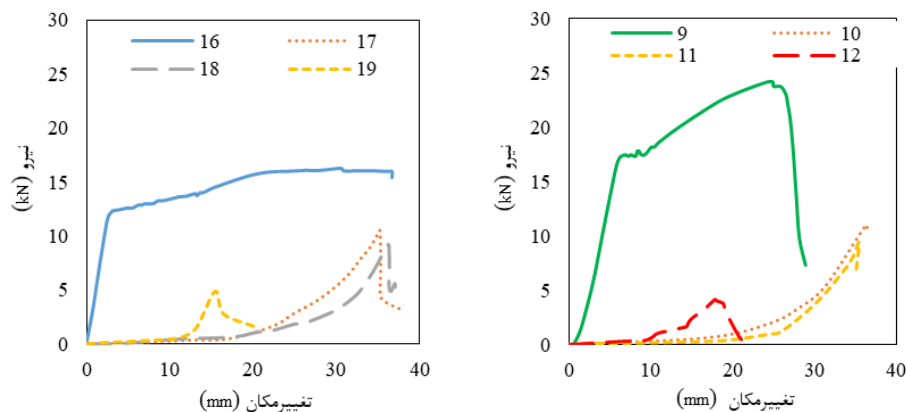
شکل ۱۵- بررسی تأثیر شرایط زنگ‌زدگی میلگرد در نتایج نمونه‌ها
