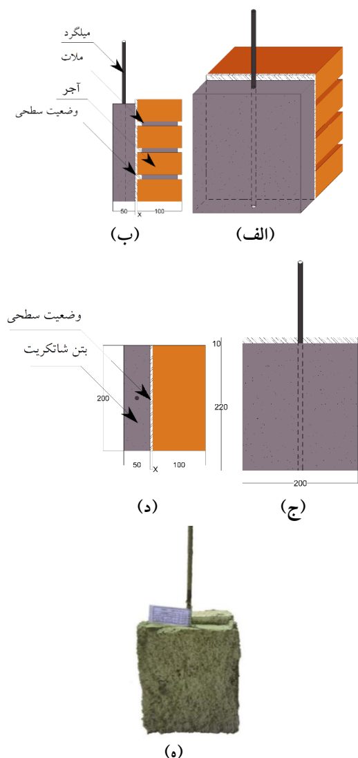
شکل ۳- مشخصات ابعادی نمونه‌ها (اندازه‌ها بر حسب میلی‌متر است): (الف) تصویر سه‌بعدی و شماتیک نمونه، (ب) تصویر شماتیک از نمای کناری نمونه، (ج) تصویر شماتیک از نمای روبه‌روی نمونه، (د) تصویر شماتیک از نمای بالای نمونه، (ه) تصویر واقعی از نمای روبه‌روی نمونه
