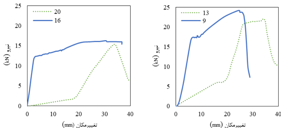
شکل ۱۶- نمودار نیرو - تغییر مکان مربوط به نمونه‌ها با وضعیت‌های سطحی متفاوت و با میلگردهای آج‌دار و ساده
