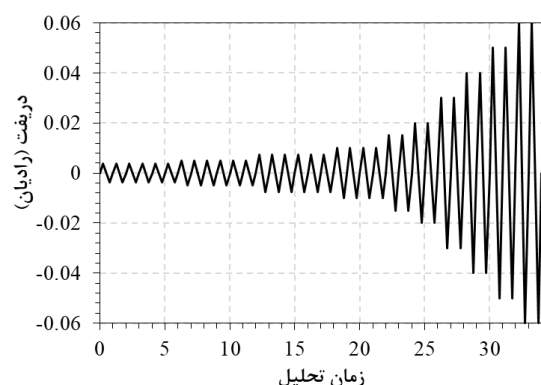
شکل ۲- تاریخچه بارگذاری مورد استفاده در تحلیل نمونه ها [۲۶]
