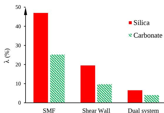
شکل ۱۱- مقادیر \lambda برای انواع سیستم‌های باربر لرزه‌ای و برای دو نوع سنگدانه، به‌ازای طول طبقات ۳،۲ متر
