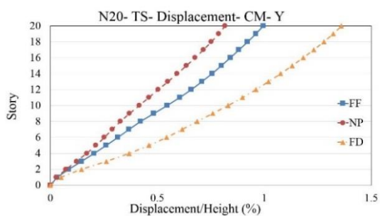
شکل ۷- نسبت جابه‌جایی طبقات به ارتفاع ساختمان برای مرکز جرم طبقات در جهت Y به ترتیب شکل‌های سمت چپ: ساختمان‌های پیچشی سخت و شکل‌های سمت راست: ساختمان‌های پیچشی نرم
