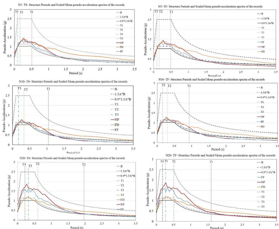
شکل ۶- طیف شبه‌شتاب میانگین رکوردهای مقیاس‌شده برای هر ساختمان؛ به‌ترتیب شکل‌های سمت چپ: ساختمان‌های پیچشی سخت و شکل‌های سمت راست: ساختمان‌های پیچشی نرم
