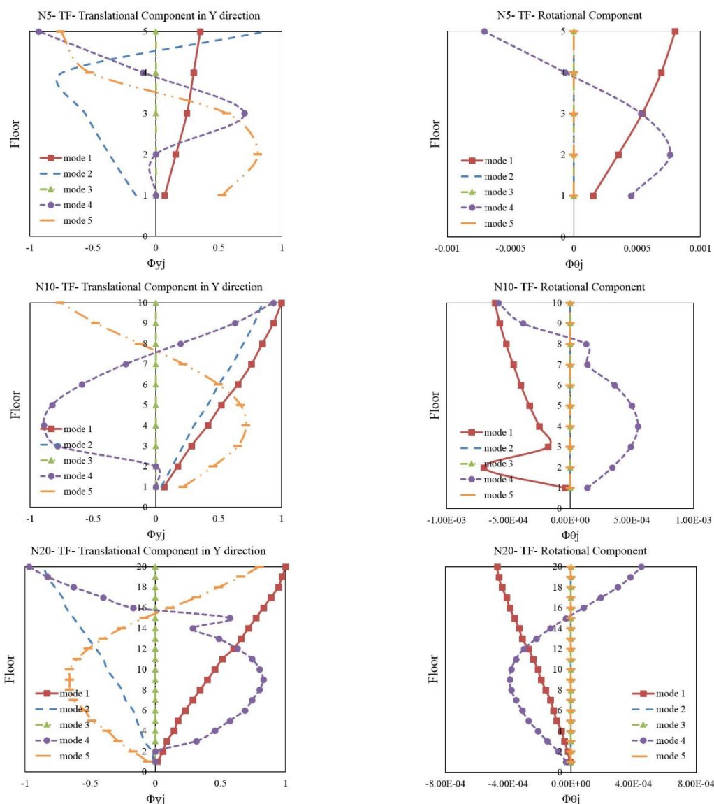
شکل ۳- شکل‌های مودی الاستیک ساختمان‌های پیش‌تنشی نرم ۵، ۱۰ و ۲۰ طبقه به‌ترتیب شکل‌های سمت چپ: مؤلفه انتقالی در جهت Y و شکل‌های سمت راست: مؤلفه دورانی
