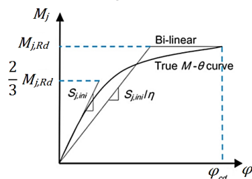
شکل ۲- نمودار لنگر-دوران اتصال ایده‌آل شده [۲۰]
