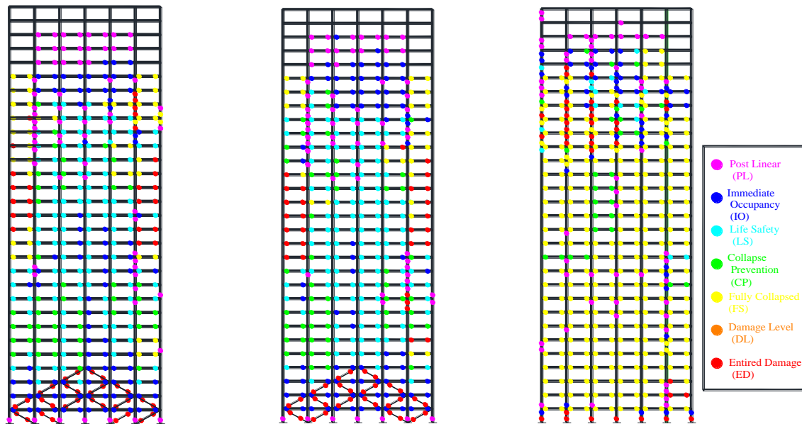
شکل ۱۴- آرایش مفاصل پلاستیک تشکیل شده در بیکره قاب صلب گوشه ای پلان و هم راستا با محور X؛ در آخرین ثانیه قبل از فروریزش کلی اسکلت مقاوم سازه تحت رکورد مقیاس شده STC (الف) مدل ۱ با اسکلت قاب خمشی محیطی پایه (ب) مدل ۲ با بیکرنبدی المان‌های زیر بزرگ مقیاس دارای اتصال دو طرفه ستون‌های تکیه گاهی (ج) مدل ۳ با بیکرنبدی المان‌های زیر بزرگ مقیاس دارای اتصال یک طرفه ستون‌های تکیه گاهی
