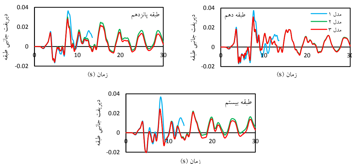
شکل ۱۲- نمودار تاریخچه زمانی دریفت طبقات دهم، پانزدهم و بیستم در نقطه A در جهت Y تحت رکورد STC: مدل ۱ با اسکلت قاب خمشی محیطی پایه (آبی)؛ مدل ۲ با اسکلت قاب خمشی محیطی دارای المان‌های زیر بزرگ مقیاس با اتصال دو طرفه به ستون‌های تکیه گاهی (سبز)؛ مدل ۳ با اسکلت قاب خمشی محیطی دارای المان‌های زیر بزرگ مقیاس با اتصال یک طرفه به ستون‌های تکیه گاهی (قرمز)
